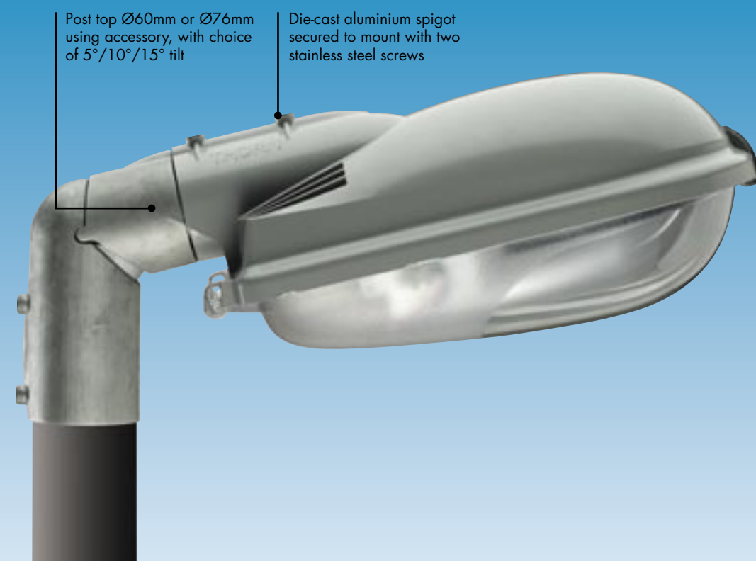
Tiltable spigot
